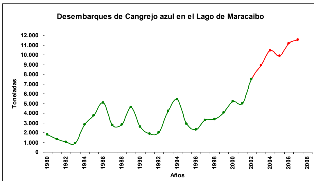
Figura 2. Desembarques anuales en toneladas de cangrejo azul, Callinectes sapidus , en el Lago de Maracaibo.
