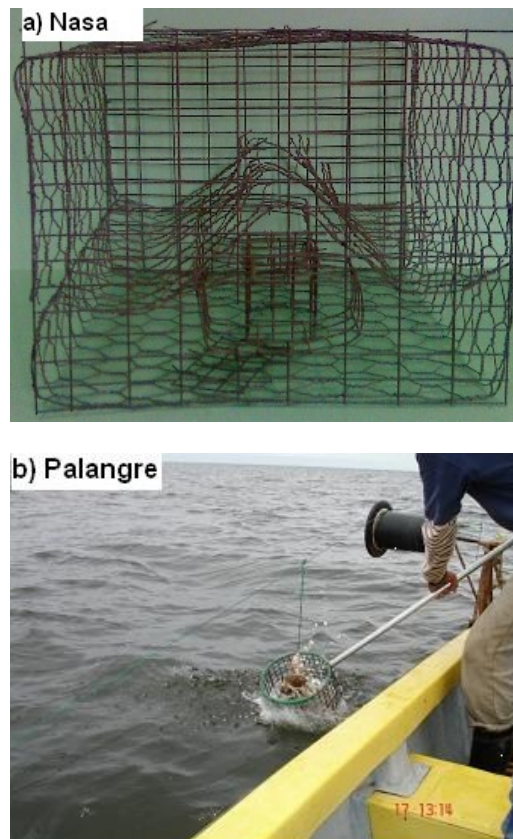
Figura 1. Artes de pesca utilizados para la captura del cangrejo azul, Callinectes sapidus , en el Lago de Maracaibo, a) Nasa y b) Palangre.
