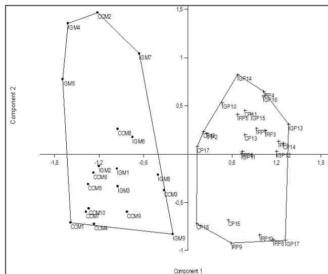
Figura 3. Análisis de componentes principales (ACP) de la densidad media de peces por transecto en manglares y pastos marinos. El eje horizontal representa el primer eje del ACP y el eje vertical el segundo eje del ACP. CC: ciénaga de Cholón; IG: Isla Grande; IR: Isla Rosario; M: manglar, P: pastos marinos. Las líneas rectas demarcan el grupo de transectos de cada hábitat. Los tres primeros ejes explicaron al menos el 54,1% de la variación de los datos (eje 1: 33,5 %, eje 2: 12,1%, eje 3: 8,6%).
